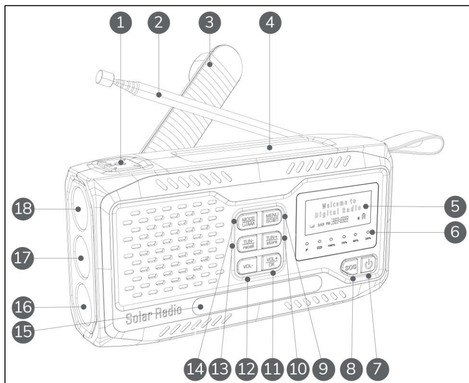
Abbildung 1: Vorderansicht.
