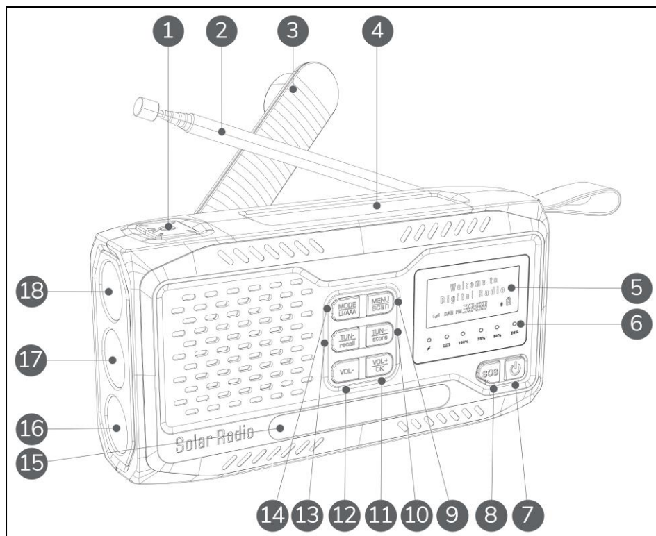
Figuur 1: Vooraanzicht.
