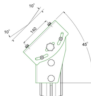
DETAIL B SCALE 0.150
